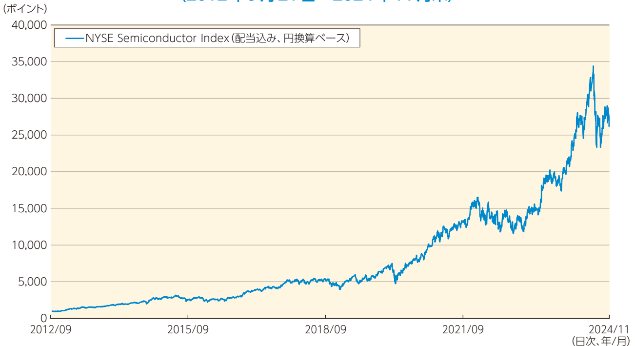
NYSE Semiconductor Index (配当込み、円換算ベース) の推移 (2012年9月21日～2024年11月末)
